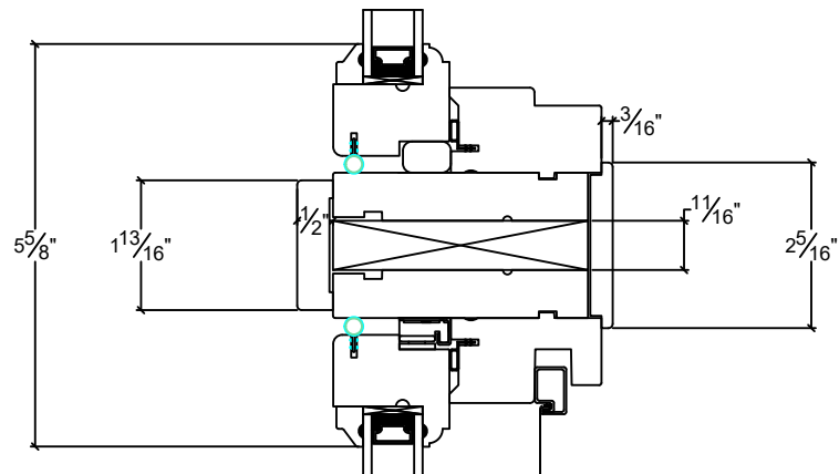
TRANSOM / CASEMENT STACK 3 9/16" JAMB C/W FILLER
