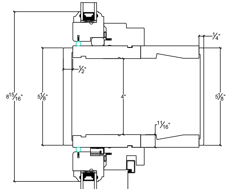
TRANSOM / CASEMENT STACK 6 9/16" JAMB C/W POCKET
