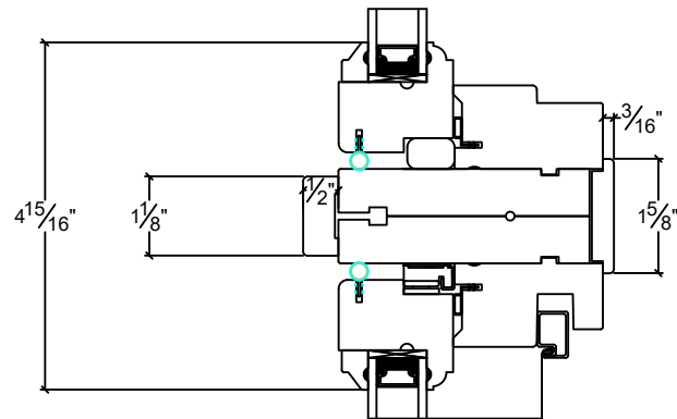
TRANSOM / CASEMENT STACK 3 9/16" JAMB
