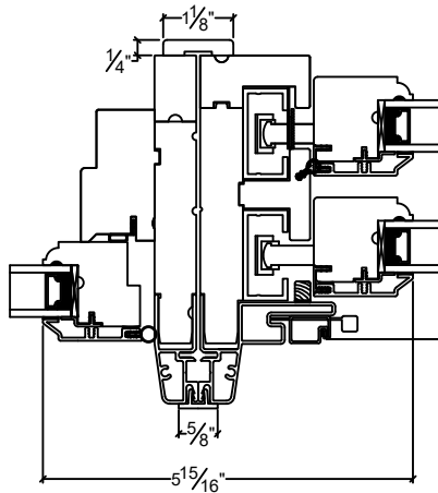
TRANSOM / DH500 CLAD MULL 4 9/16" JAMB
