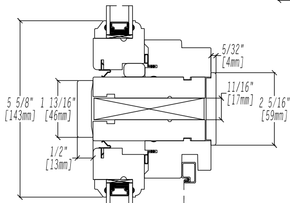
TRANSOM / AWNING STACK 3 9/16" JAMB C/W FILLER
