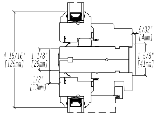
TRANSOM / AWNING STACK 3 9/16" JAMB
