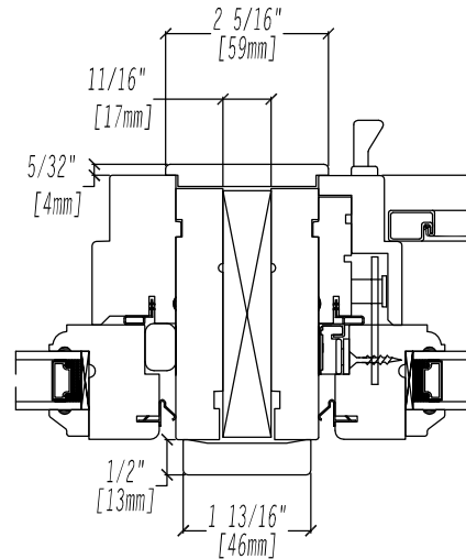
TRANSOM / AWNING MULL 3 9/16" JAMB C/W FILLER
