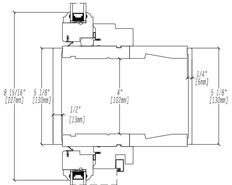
TRANSOM / AWNING STACK 6 9/16" JAMB C/W POCKET
