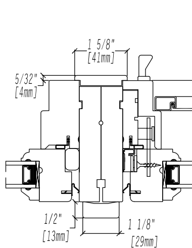
TRANSOM / AWNING MULL 3 9/16" JAMB
