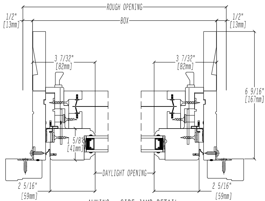
AWNING - SIDE JAMB DETAIL
