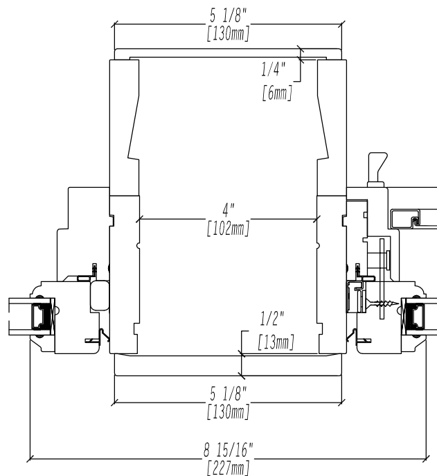
TRANSOM / AWNING MULL 6 9/16" JAMB C/W POCKET
